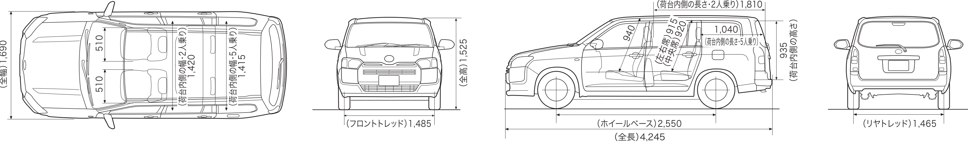
寸法図 F（ハイブリッド車） [単位：mm]
