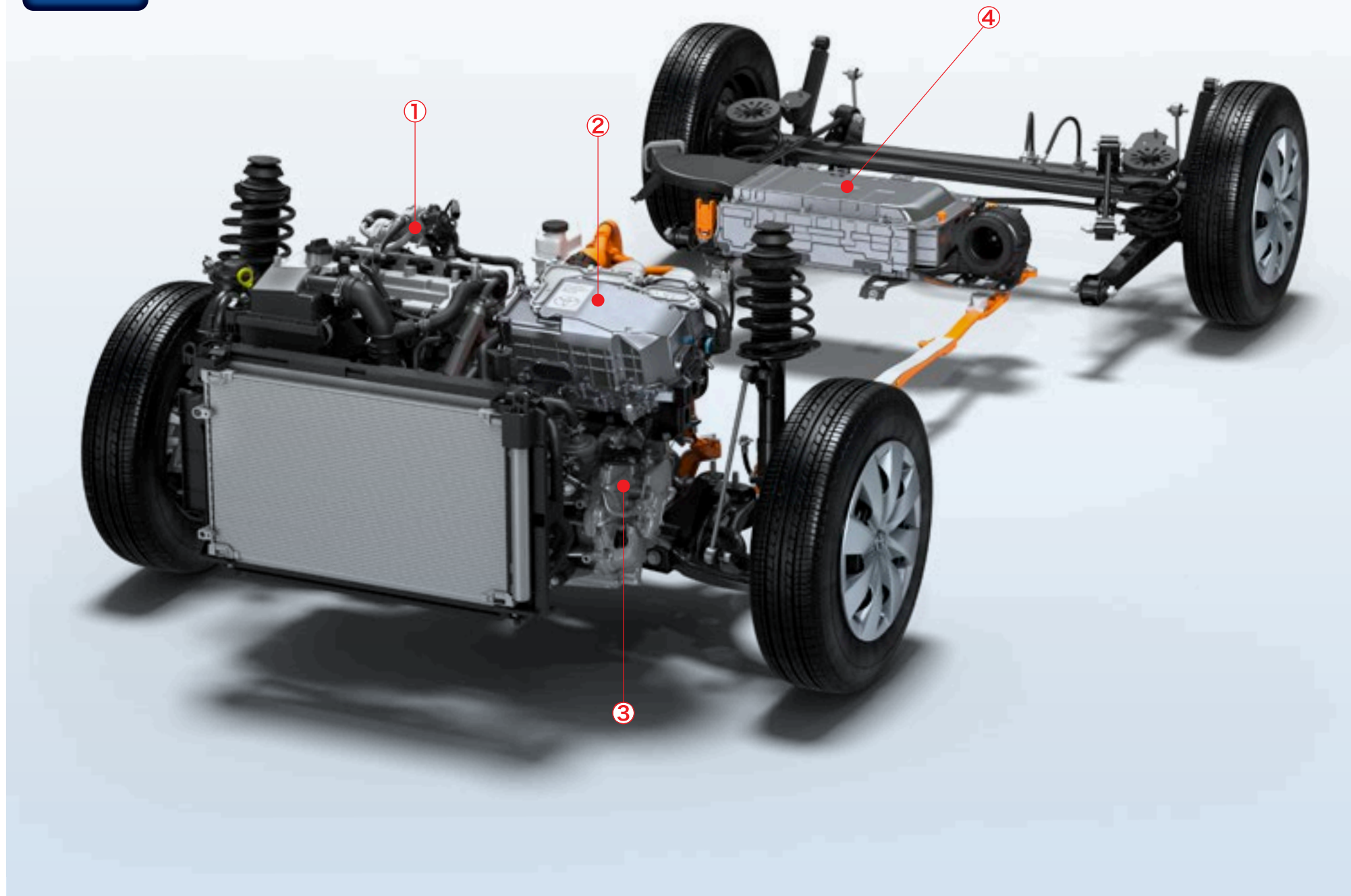
ハイブリッドシステムイメージ図
