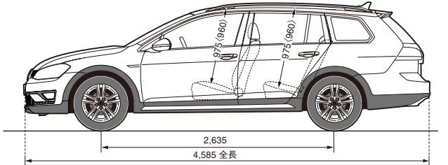
四面図 (mm)
