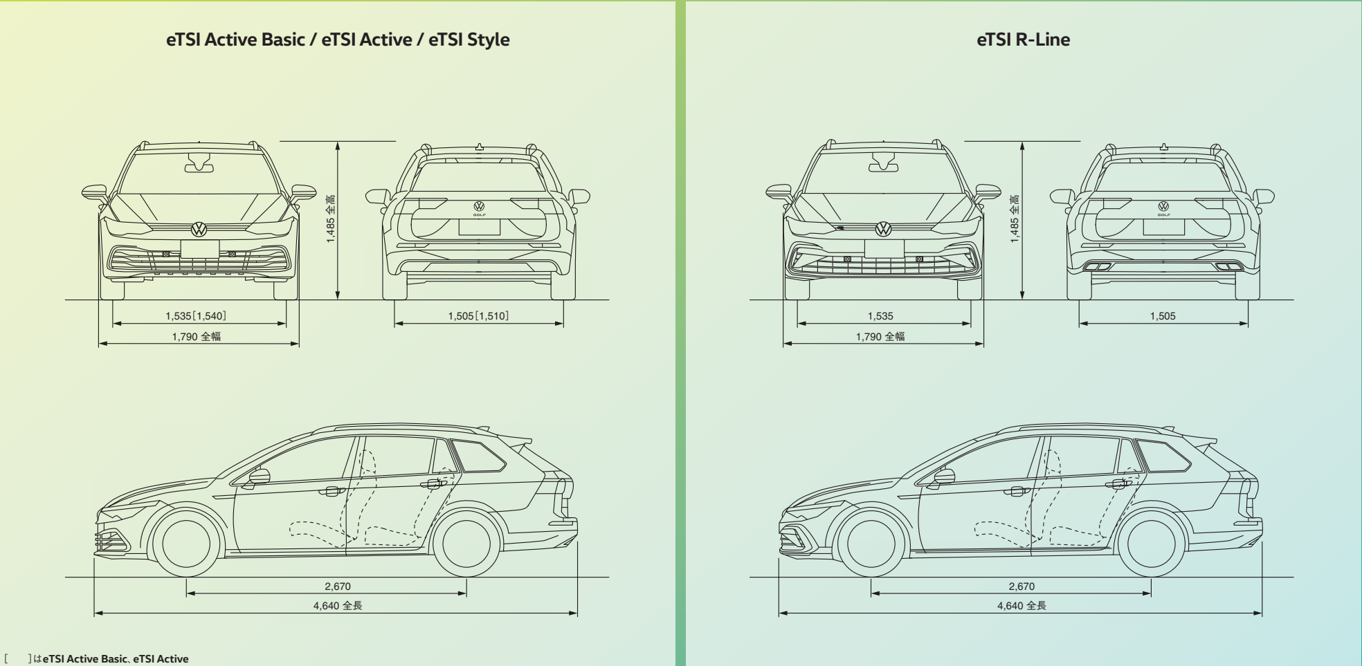
三面図 (mm)
