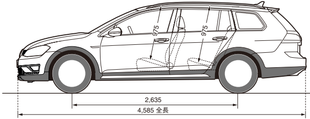
四面図(mm)
