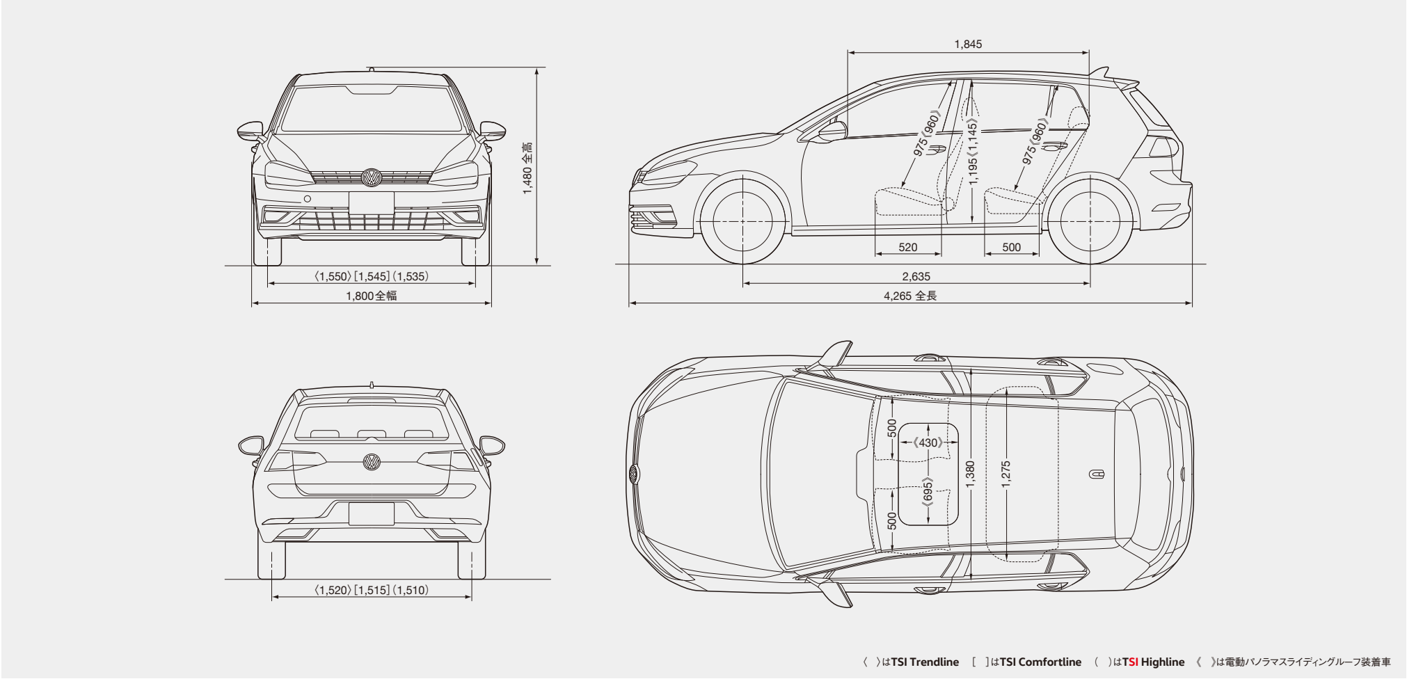
四面図(mm)
