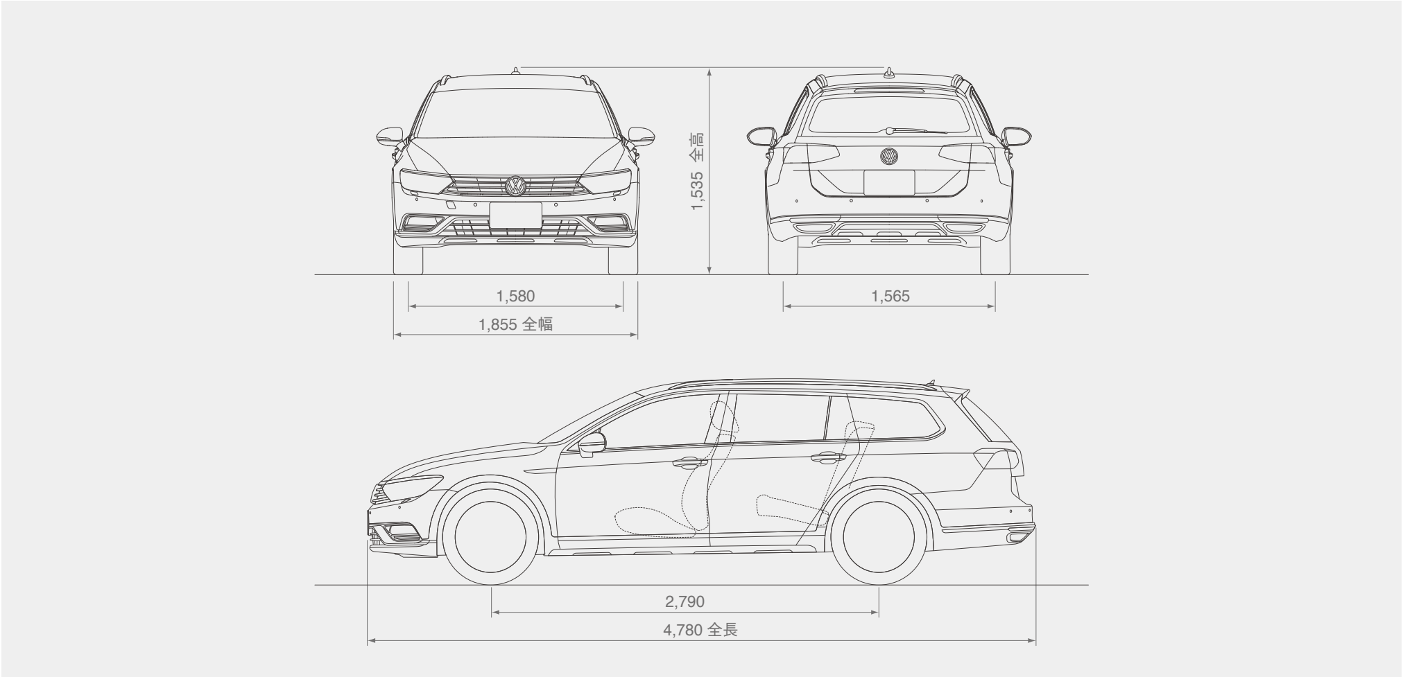
三面図(mm)
