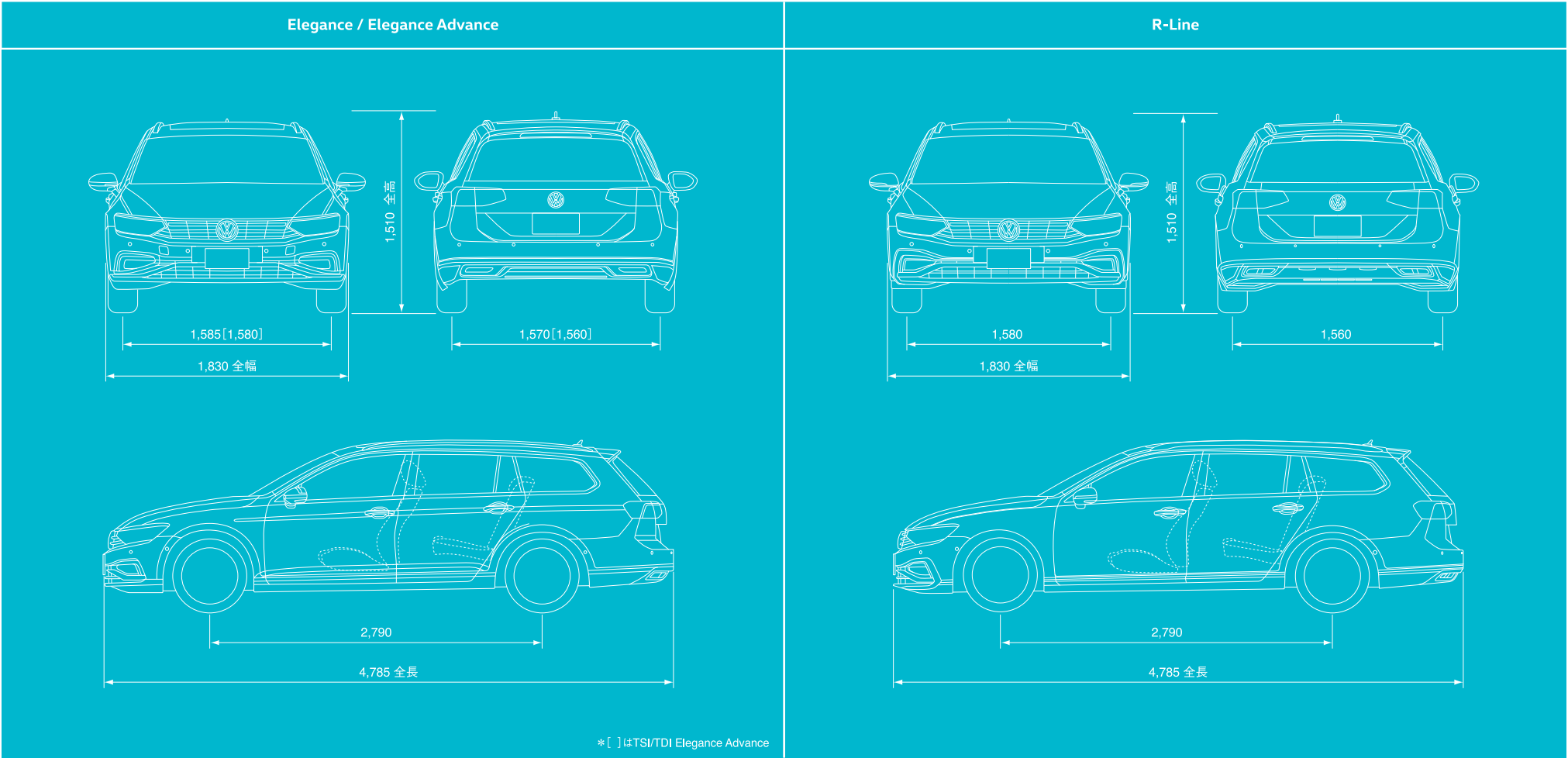
三面図(mm)
