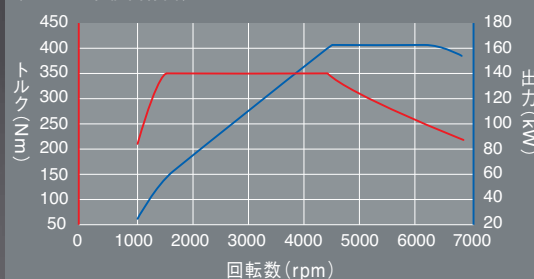
〈エンジン性能曲線図〉
