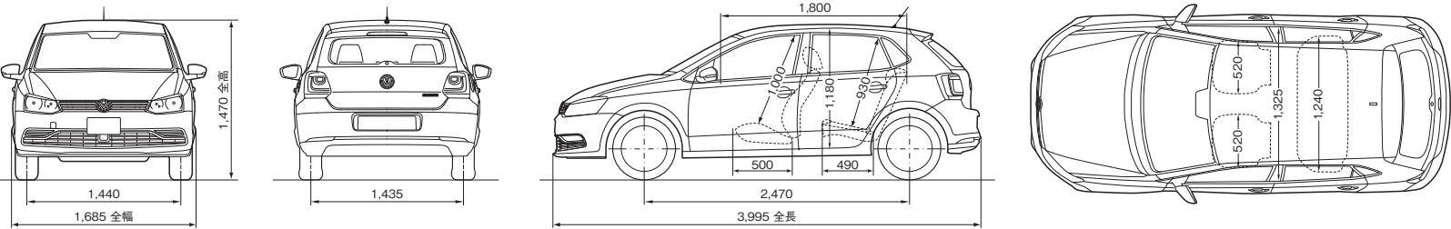
四面図 (mm)
