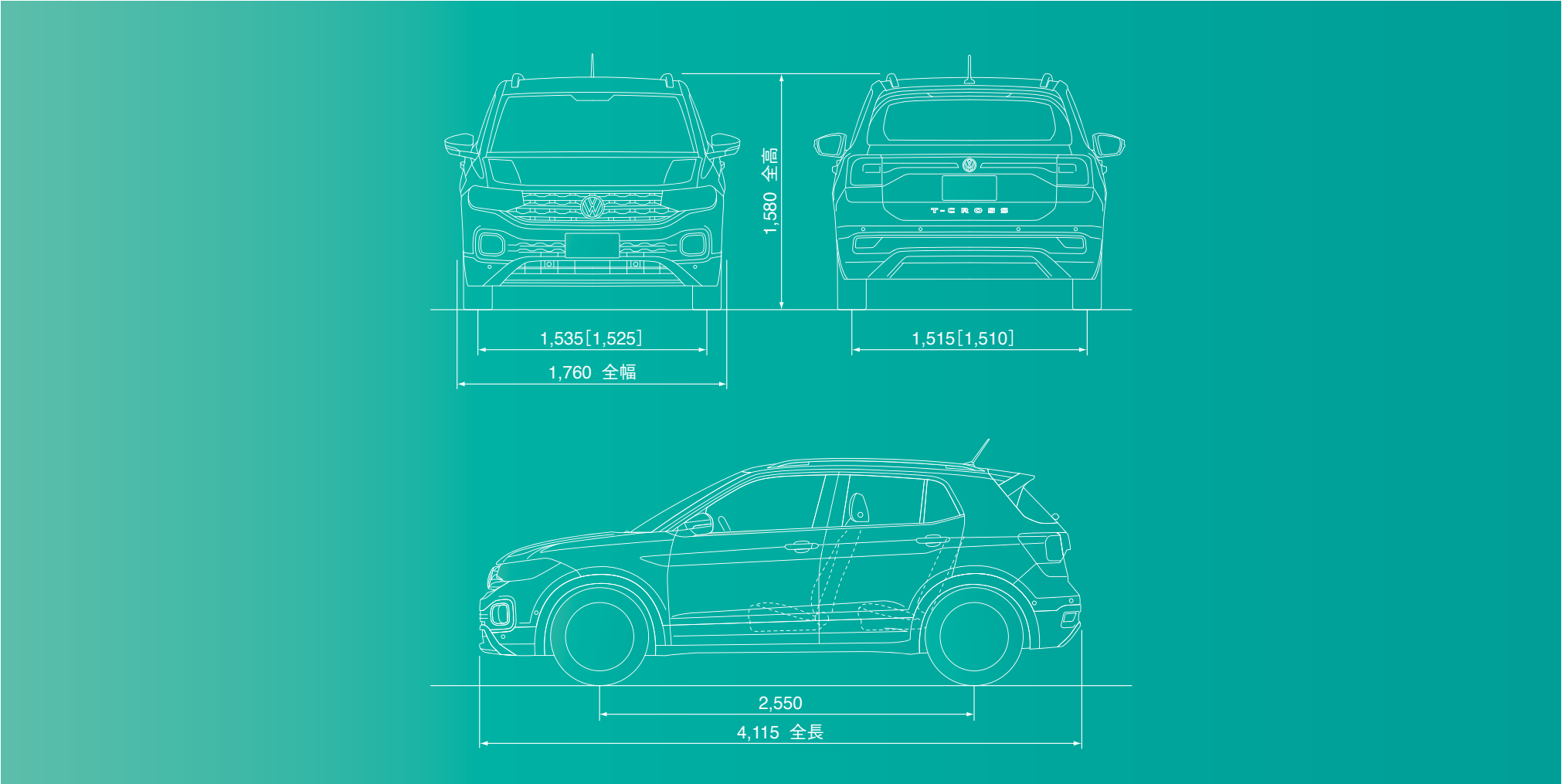
三面図(mm)
