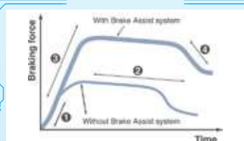
ប្រព័ន្ធដំនួយប្រឆាំងសុវត្ថិភាព BA ប្រព័ន្ធបែងចែកកម្លាំងសម្ពាធប្រឆាំង (EBD)
