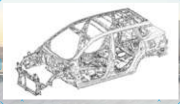
គ្រោងឆ្នាំង TNGA រឹងមាំជាងមុន 60% បត់បែន និងមានលំនឹងល្អក្នុងការប្រតិបត្តិការ
