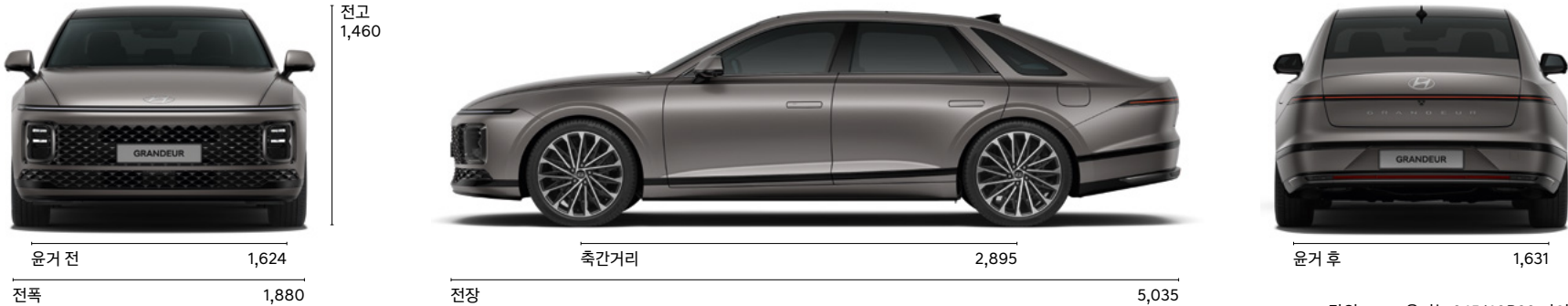
단위: mm, 윤거는 245/40R20 타이어 기준
