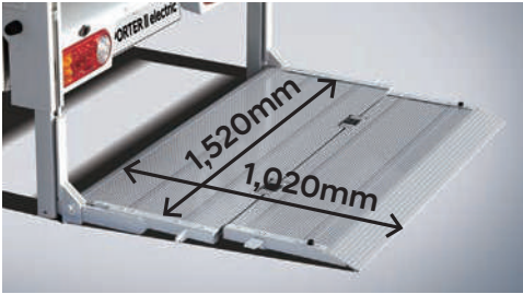
전동유압식 리프트 시스템 (허용하중 : 600kg)
