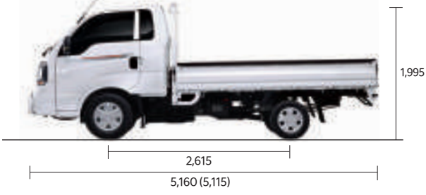
※ ( ) : 범퍼가드 미장착 사양 기준 ※ 1톤 초장축 킹캡 기준(단위 : mm)
