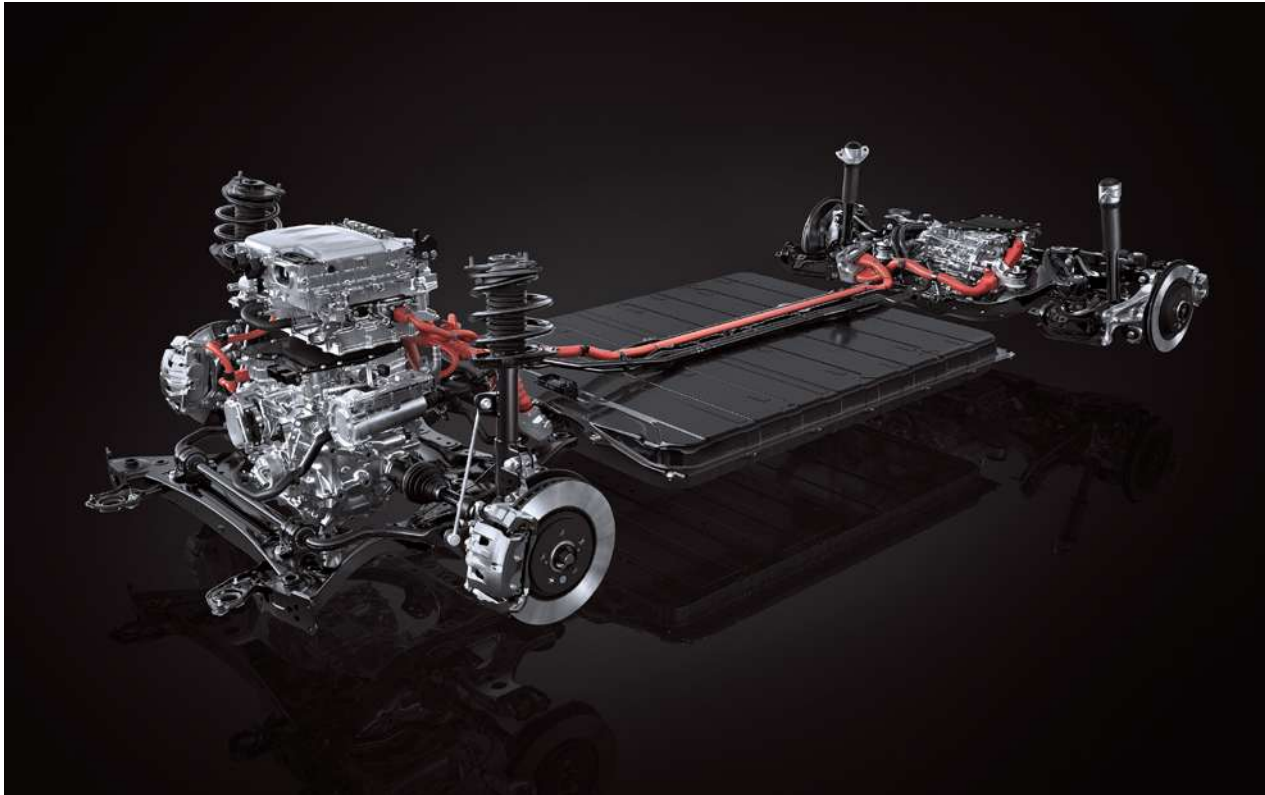
프런트 이엑슬(eAxle)
