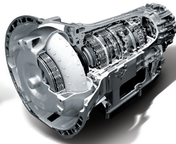
T-Tronic 5단 자동변속기
