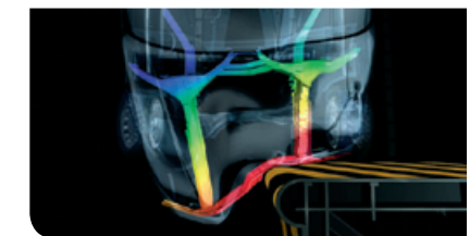
피라미드식 차체 구조
