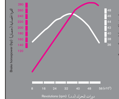
منحنى أداء محرك TB48DE (SAE Gross) TB48DE engine performance curve (SAE Gross)
