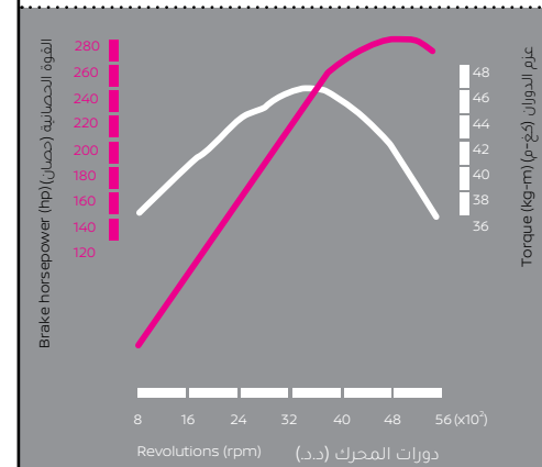
منحنى أداء محرك TB48DE (SAE Gross) TB48DE engine performance curve (SAE Gross)
