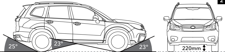
أدنى خلوص للطريق Minimum Road Clearance زاوية الاقتراب Approach Angle زاوية التخطي Break-over Angle زاوية الإقلاع Departure Angle
