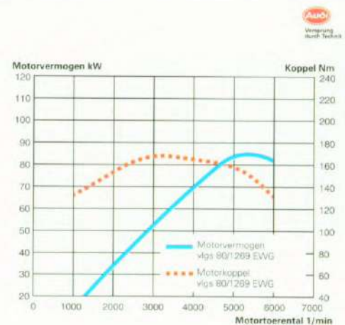
De prestaties van de 85 kW motor.
