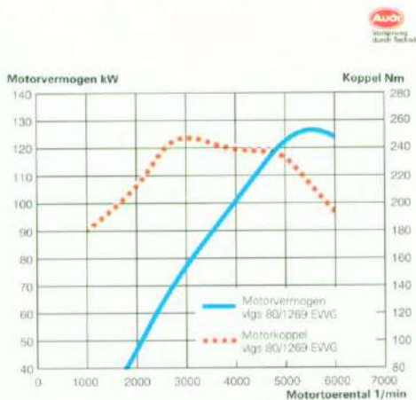
Het vermogen van de 128 kW motor.
