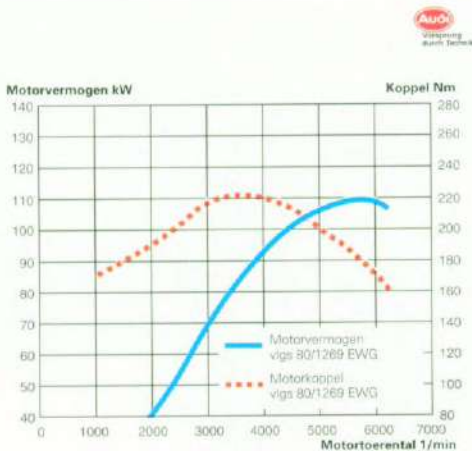
Het vermogen van de 110 kW motor.
