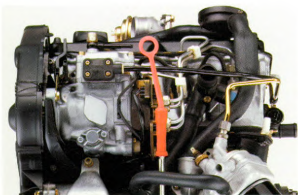
De viercilinder turbodiesel met een inhoud van 1,9 liter, 66 kW(90 pk), directe inspuiting, interkoeler en elektronisch gestuurde inspuitpomp.
