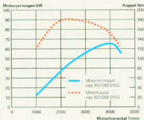
De prestaties van de 66 kW motor.
