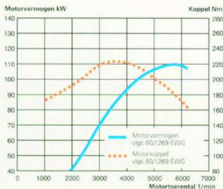
De prestaties van de 110 kW motor.
