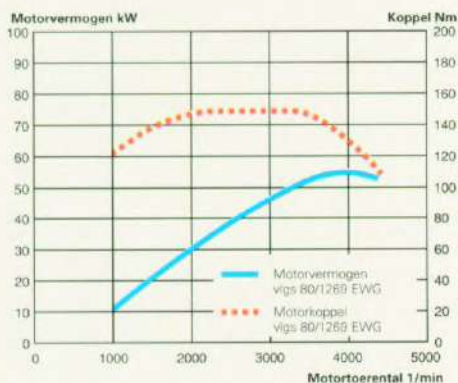
De prestaties van de 55 kW motor.
