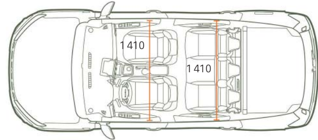
BOVENAANZICHT 5 ZITPLAATSEN
