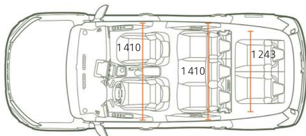
BOVENAANZICHT 7 ZITPLAATSEN
