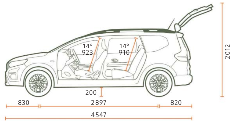
ZIJAANZICHT 5 ZITPLAATSEN
