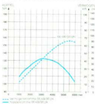
De 1.6i-16V DOHC motor met 90 pk.
