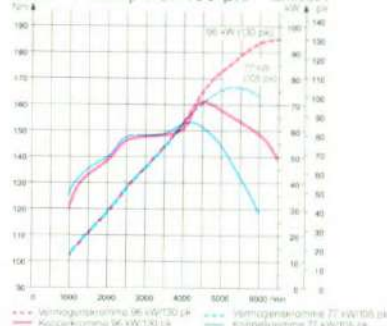
De 1.8i-16V DOHC motoren met 105 pk en 130 pk.
