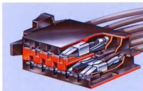
Nieuwe stekkerverbindingen.
