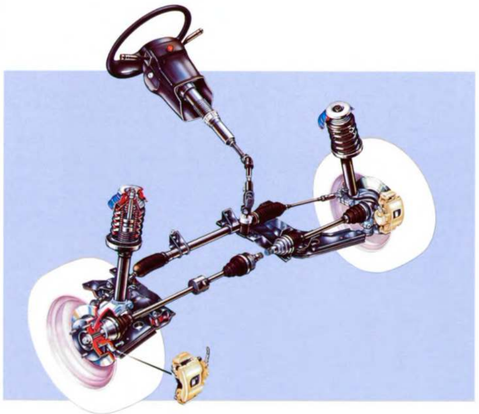
De voorwielophanging en stuurinrichting
