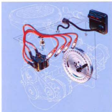
Verdelerloos ontstekingsysteem.
