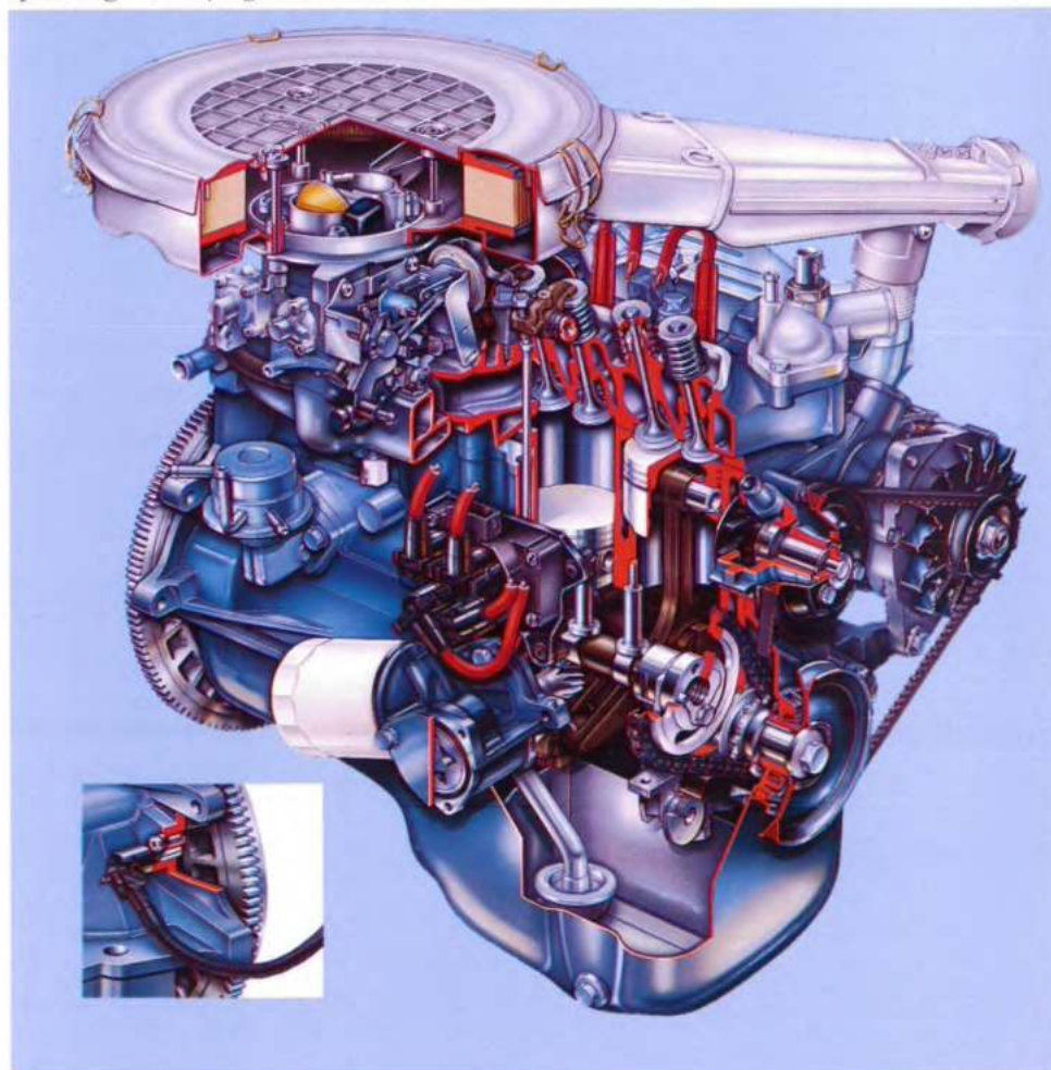
Afbeelding van de opengewerkte 1.1 HCS motor.
