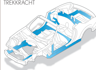
VEILIGHEIDSKOOI UIT STAAL MET HOGE TREKKRACHT
