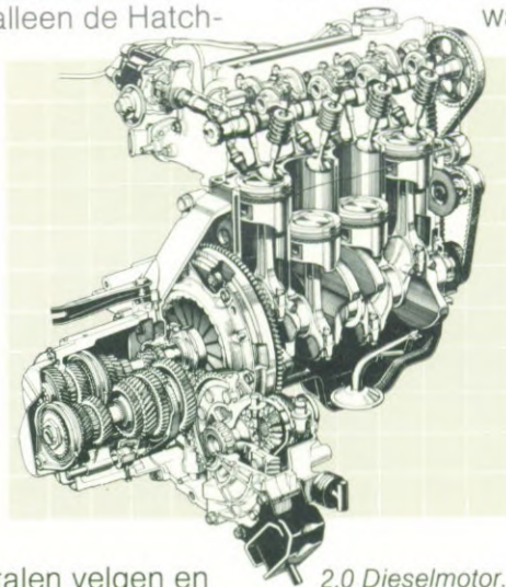
2.0 Dieselmotor.
