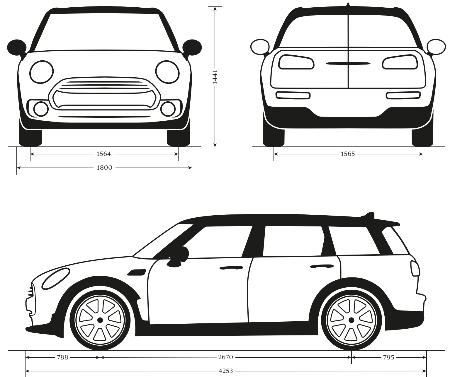
Spoorbreedte Cooper S: 1560 vóór, 1561 achter. Alle maten in mm.
