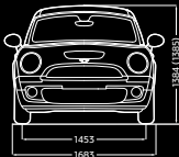
Alle afmetingen in mm.
