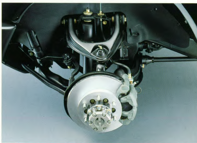
Onafhankelijke voorwielophanging met wishbone en torsiestang, en geventileerde schijfremmen.
