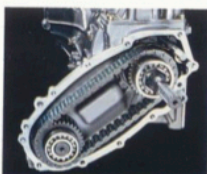
Een sterke en soepele ketting brengt een stille overgang naar vierwiel-aandrijving tot stand.
