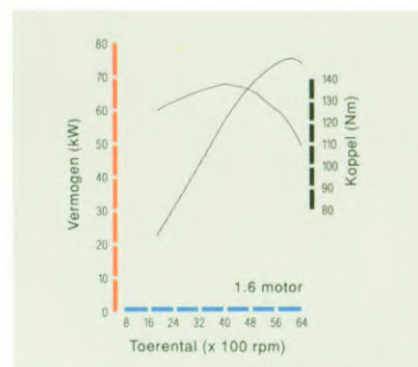
Vermogens- en koppelkromme
