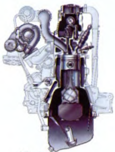
Nieuwe precisietechnieken zorgen voor een betere regeling van het brandstofverbruik, waardoor de ECOTEC-motoren bij lage toerentallen al een hoog koppel bereiken, en dus uitzonderlijk zuinig zijn.
