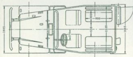
Kort chassis
