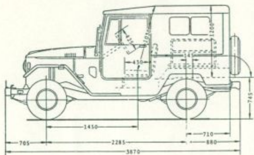
Kort chassis
