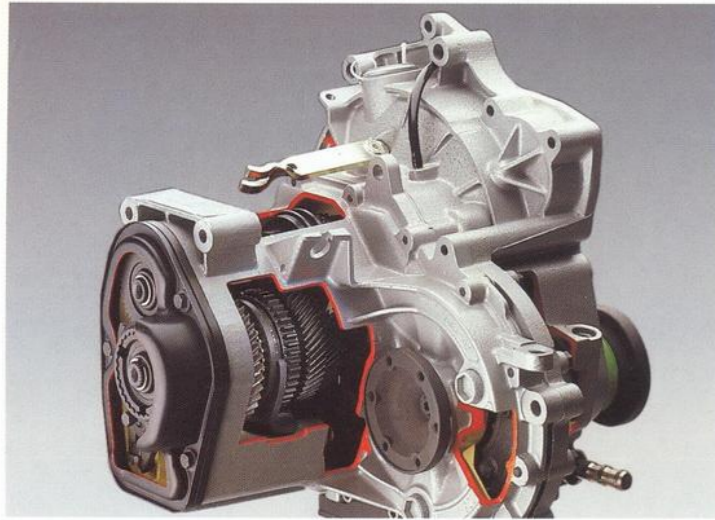
De 4+E versnellingsbak Met de vijf versnellingen, die u hiermee tot uw beschikking heeft, kunt u het toerental van de motor verlagen, waardoor een lager geluidsniveau, een lager brandstofverbruik en minder slijtage optreedt.
