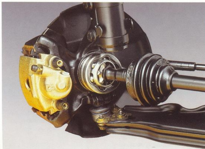
De schijfremmen De schijfremmen op de vooras met grote asbestvrije remblokken garanderen u een zekere remwerking, een optimaal remvermogen en een lange levensduur.
