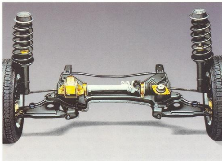
De McPherson-voorwielophanging Mede door deze voorwielophanging kenmerkt uw auto zich door een uitstekende wegligging, een hoog rij-comfort en een lichte besturing. In combinatie met de zelfcorrigerende stuurinrichting blijft uw auto koersvast. Zelfs als u remt met een van de voorwielen op een onverharde ondergrond.
