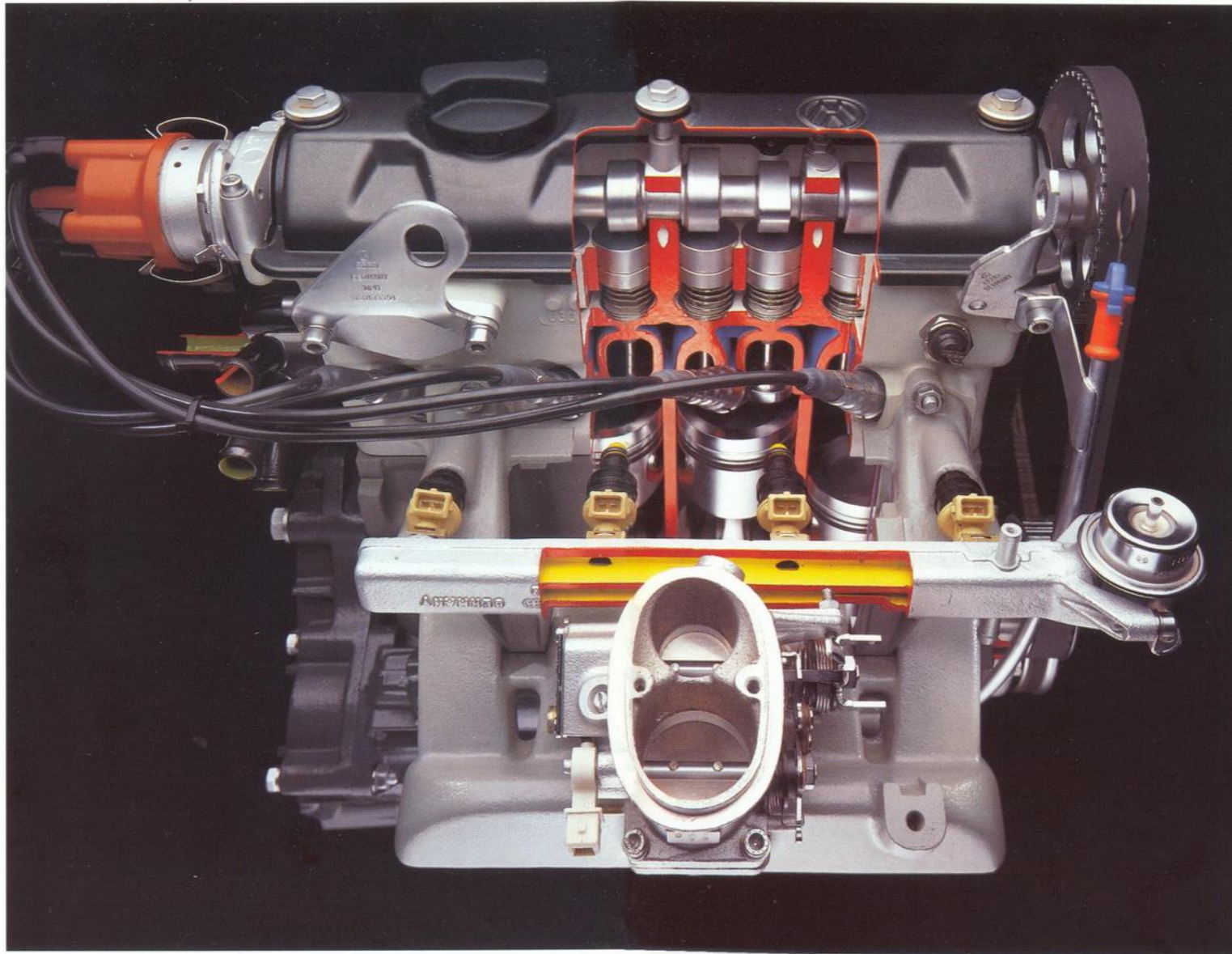
De digijet-motor Deze elektronisch geregelde injectie-motor is bijzonder schoon door z'n geregelde katalysator met lambda-regeling. Bijzonder kenmerk van deze motor is een hoog koppel bij een laag toerental.
