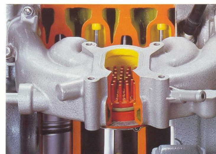
De elektronische mengselvoorverwarming "Egel" Bij een koude start zorgt de elektronisch verwarmde "egel" voor een voorverwarming van het brandstof-lucht-mengsel, hetgeen van positieve invloed is op het snel rustig stationair draaien van de motor en daardoor ook op het brandstofverbruik.
