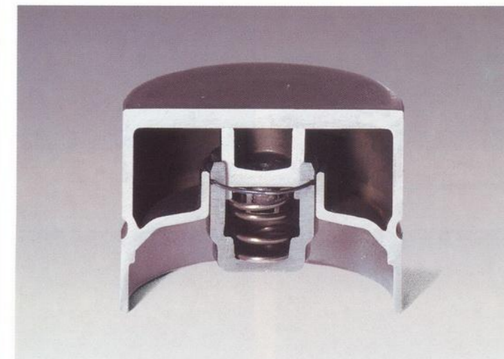
De hydraulische klepstoters Deze klepstoters zijn onderhoudsvrij. Ze zorgen bij praktisch elke nokkenas-omwenteling voor een juiste bediening van de kleppen, met alle voordelen vandien.
