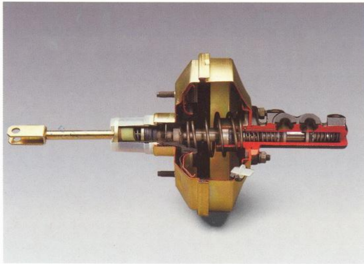
De rembechtiger Met slechts weinig druk op uw rempedaal brengt u uw auto rustig tot stilstand. De door de motor in het inlaatspruitstuk opgebouwde onderdruk wordt door de rembechtiger gebruikt ter ondersteuning van de rempedaaldruk.
