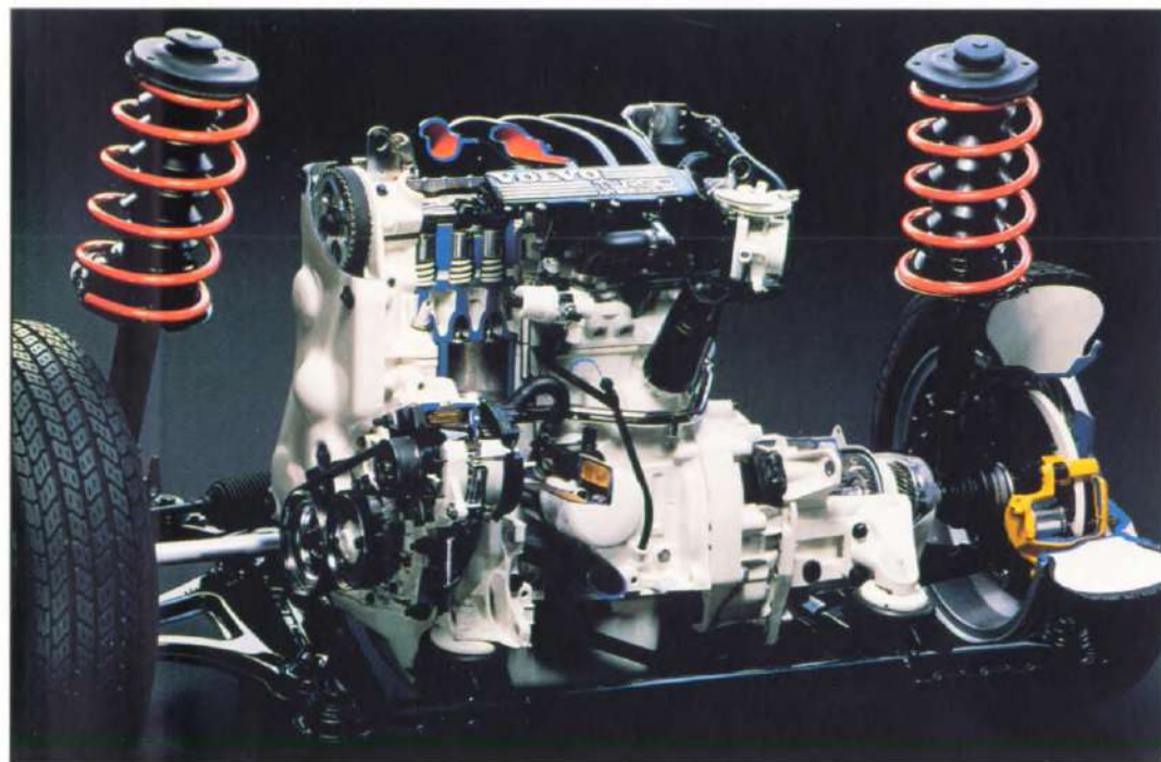
De voorwielophanging is onafhankelijk met MacPherson-veerelementen, dwarsgeplaatste onderste wiendraagarmen, schroefveren en een direct werkende stabilisator.
