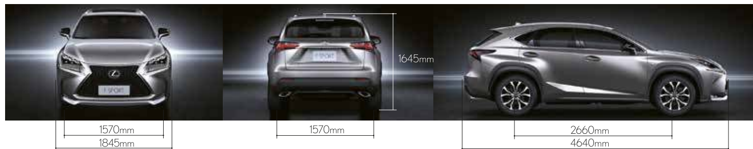
Note : Dimension of NX 300h F SPORT (mm) ; มิติของรถ NX 300h F SPORT
