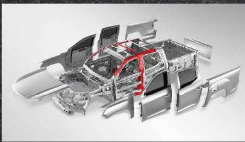
โครงสร้างตัวถังนิรภัย FSF (FULL SPACE FRAME)
