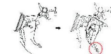
煞車踏板潰縮安全裝置
