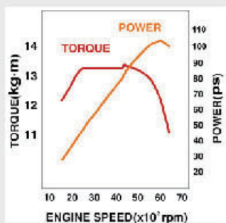
引擎性能線性圖
