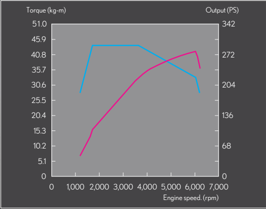
NX 350 引擎動力輸出曲線圖
