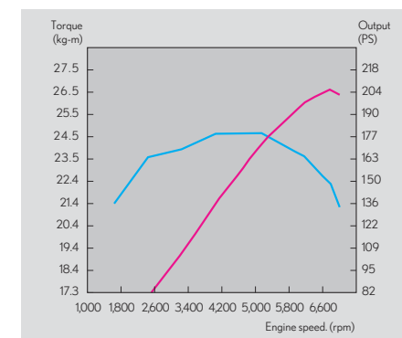
NX 250 引擎動力輸出曲線圖
