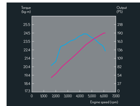
NX 350h 引擎動力輸出曲線圖
