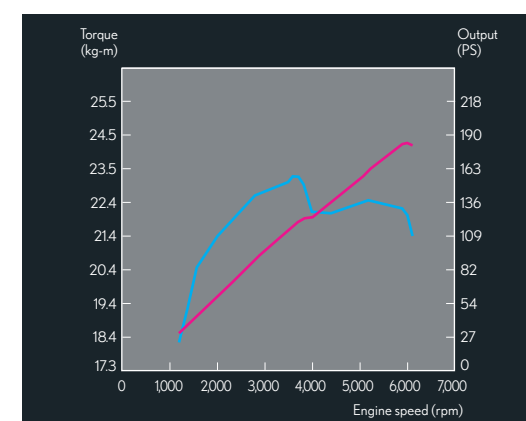
NX 450h+ 引擎動力輸出曲線圖
