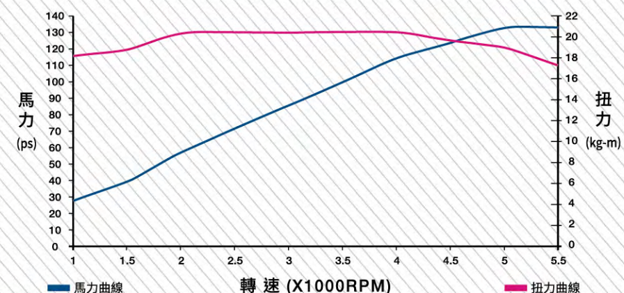
引擎性能曲線圖
