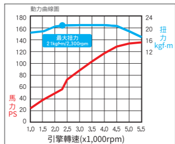
動力曲線圖
