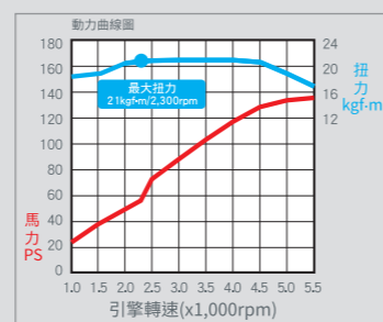
動力曲線圖
