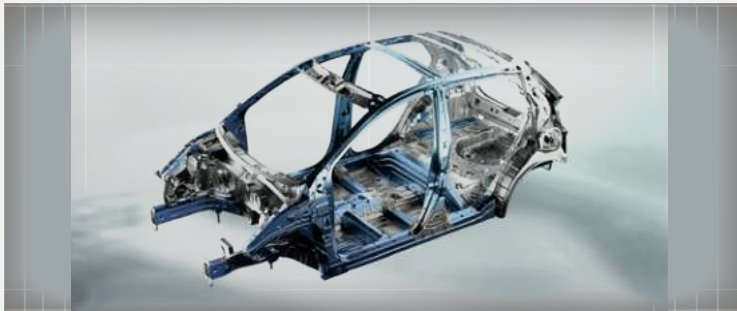
KHUNG GẮM MỎI - TĂNG TỈ LỆ THÉP CƯỜNG LỰC Cải thiện độ bền kéo 12% so với sản phẩm hiện hữu, gia tăng độ chắc chắn cho khung xe
