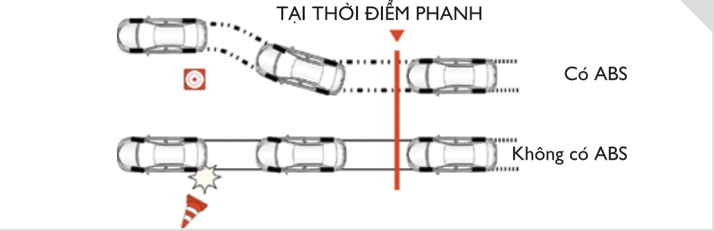
HỆ THỐNG CHỐNG BÓ CỨNG PHANH - ABS Khi được kích hoạt bằng cách đạp phanh dứt khoát, hệ thống chống bó cứng phanh ABS sẽ tự động nhấp nhả phanh liên tục, giúp các bánh xe không bị bó cứng, cho phép người lái duy trì khả năng điều khiển xe tránh chướng ngại vật và đảm bảo ổn định thân xe.
