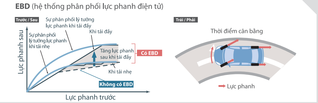
HỆ THỐNG PHÂN PHỐI LỰC PHANH ĐIỆN TỬ - EBD Phân bổ lực phanh hợp lý lên các bánh xe, giúp nâng cao hiệu quả phanh, đặc biệt khi xe đang chất tải và vào cua.
