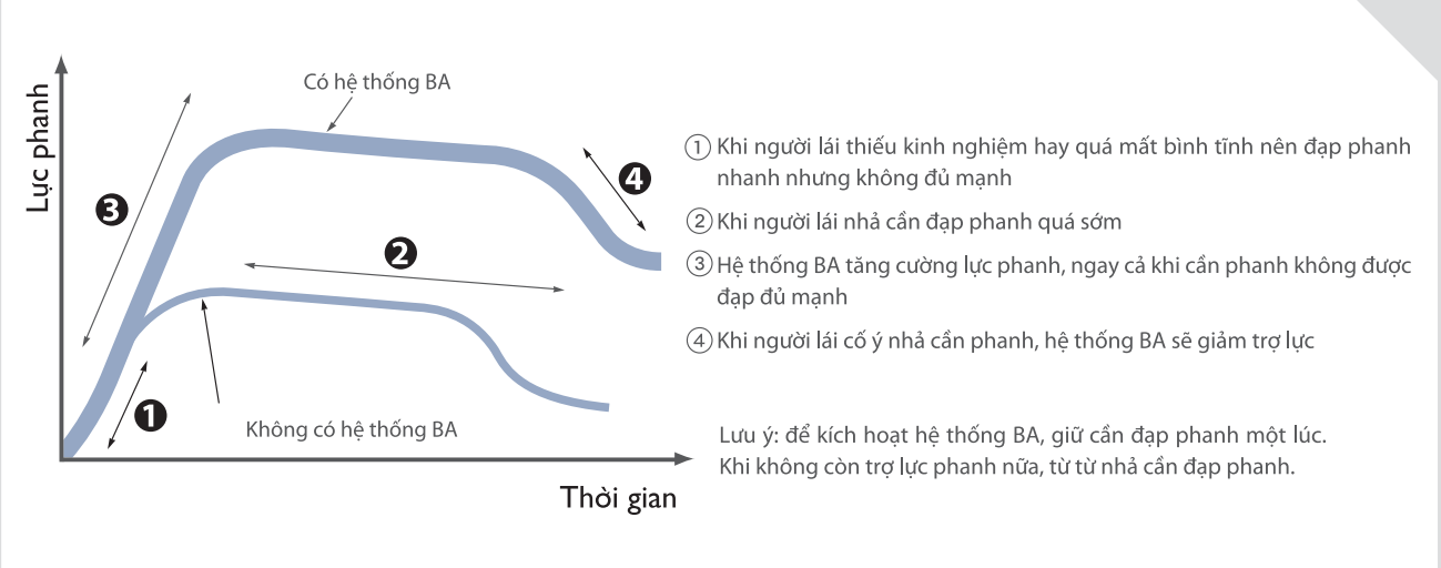
HỆ THỐNG HỖ TRỢ LỰC PHANH KHẨN CẤP - BA Tự động gia tăng thêm lực phanh trong trường hợp khẩn cấp, giúp người lái tự tin xử lý các tình huống bất ngờ.
